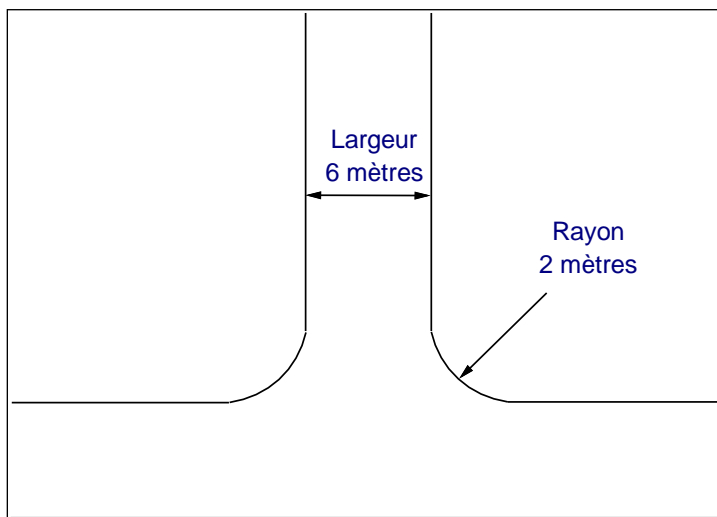
Figure 16.3.4 : Géométrie
