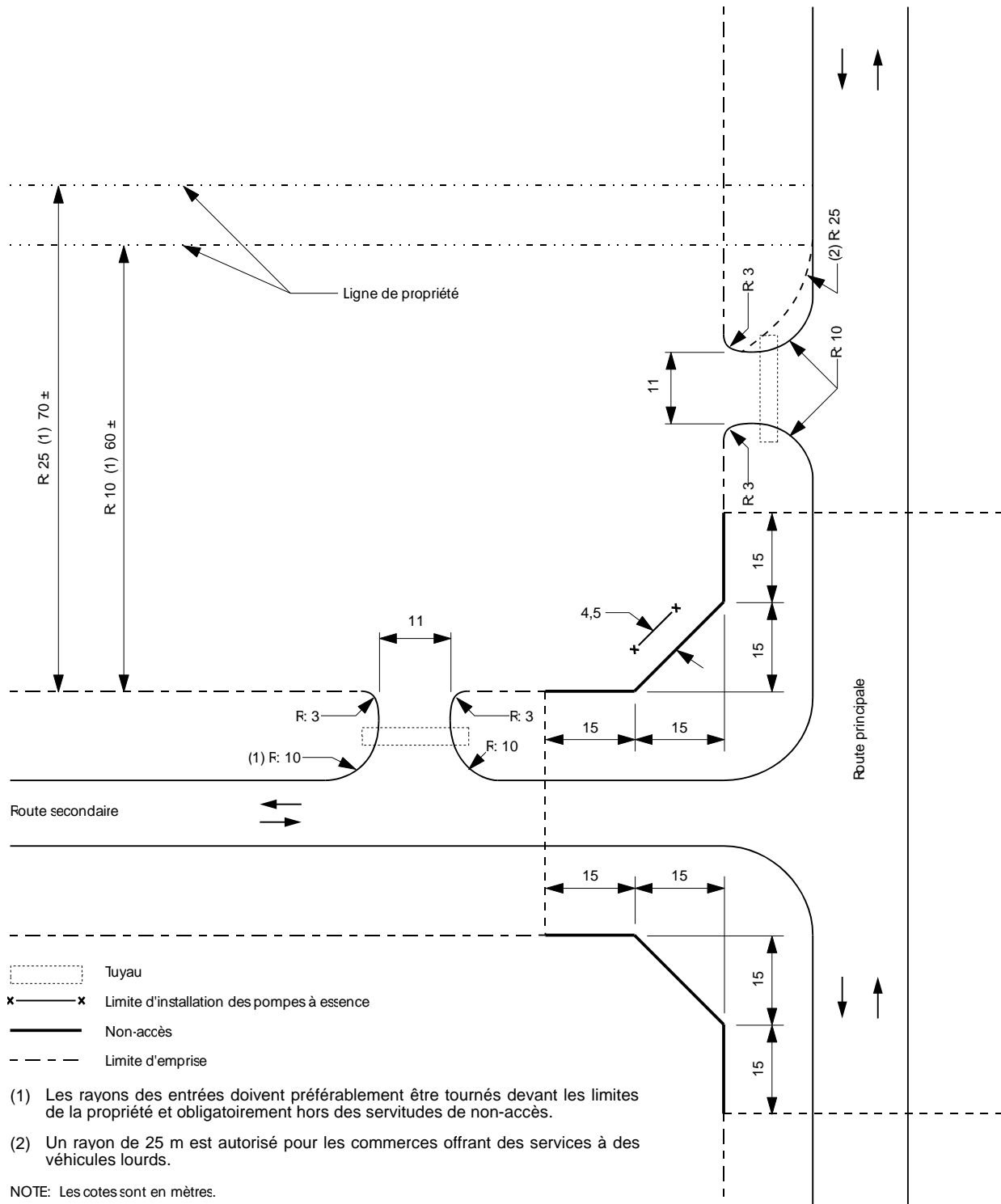
Figure 16.4.4a : Entrée commerciale à une intersection
