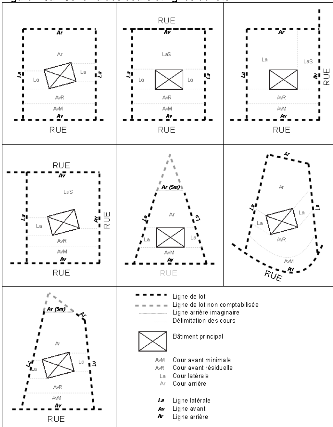
Figure 2.8a : Schéma des cours et lignes de lots
